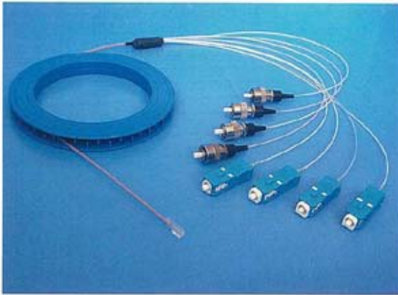
片端アレイ付きHGコード
